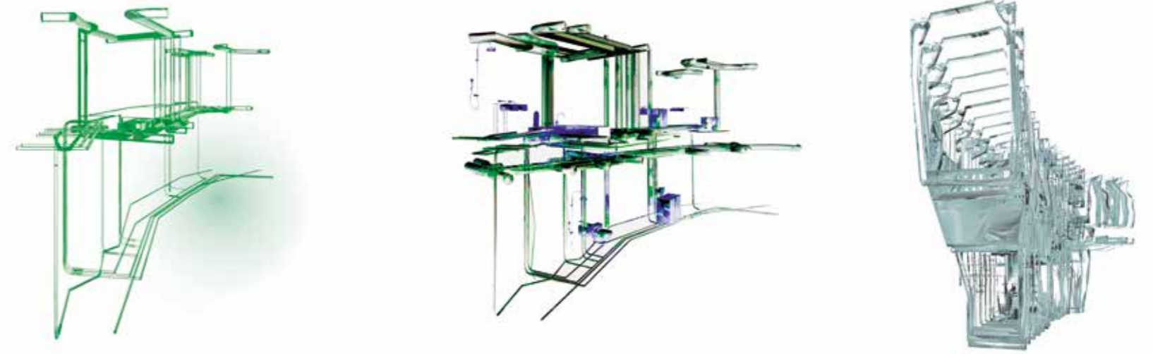
Modello 3D di studio dell'armatura 3D study model of the armature
