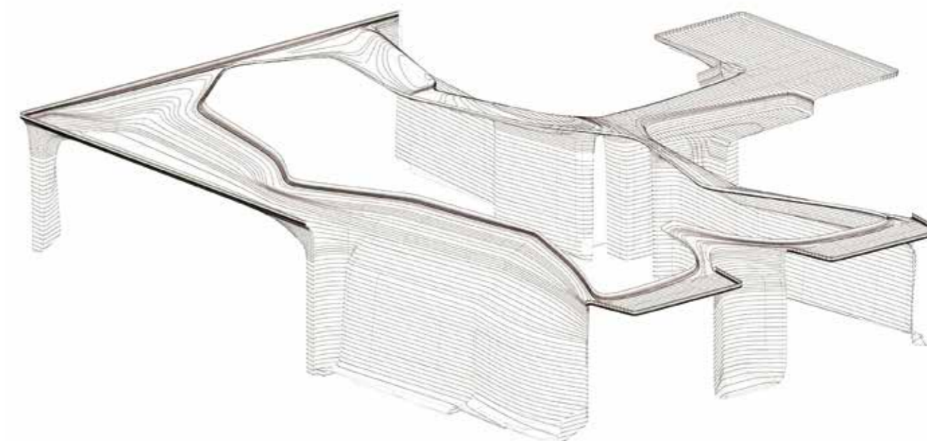
Modello 3D della superficie interna 3D model of the "lining"
